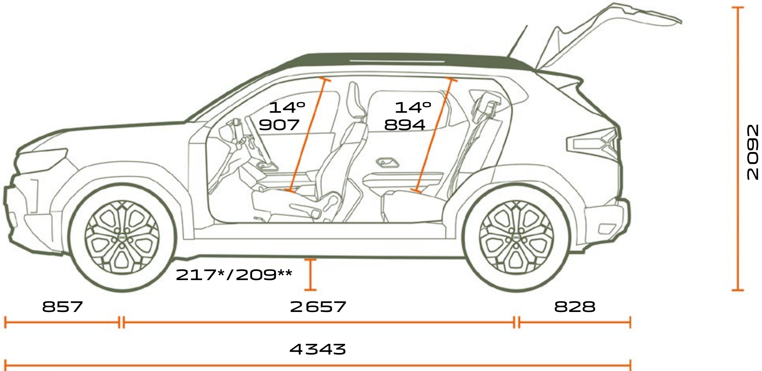
СТРАНИЧЕН ПОГЛЕД
