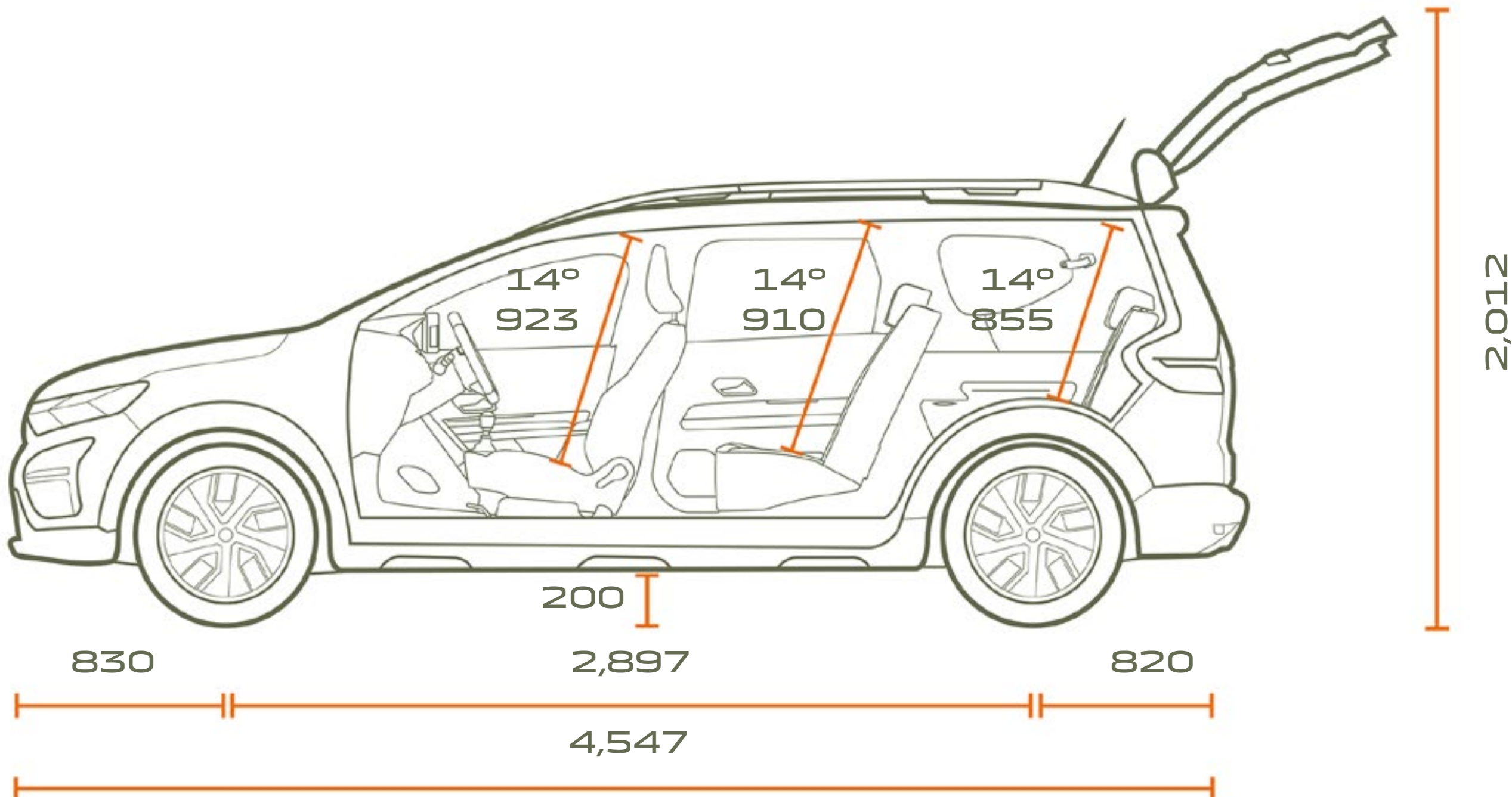
СТРАНИЧЕН ПОГЛЕД НА 7 СЕДИШТА
