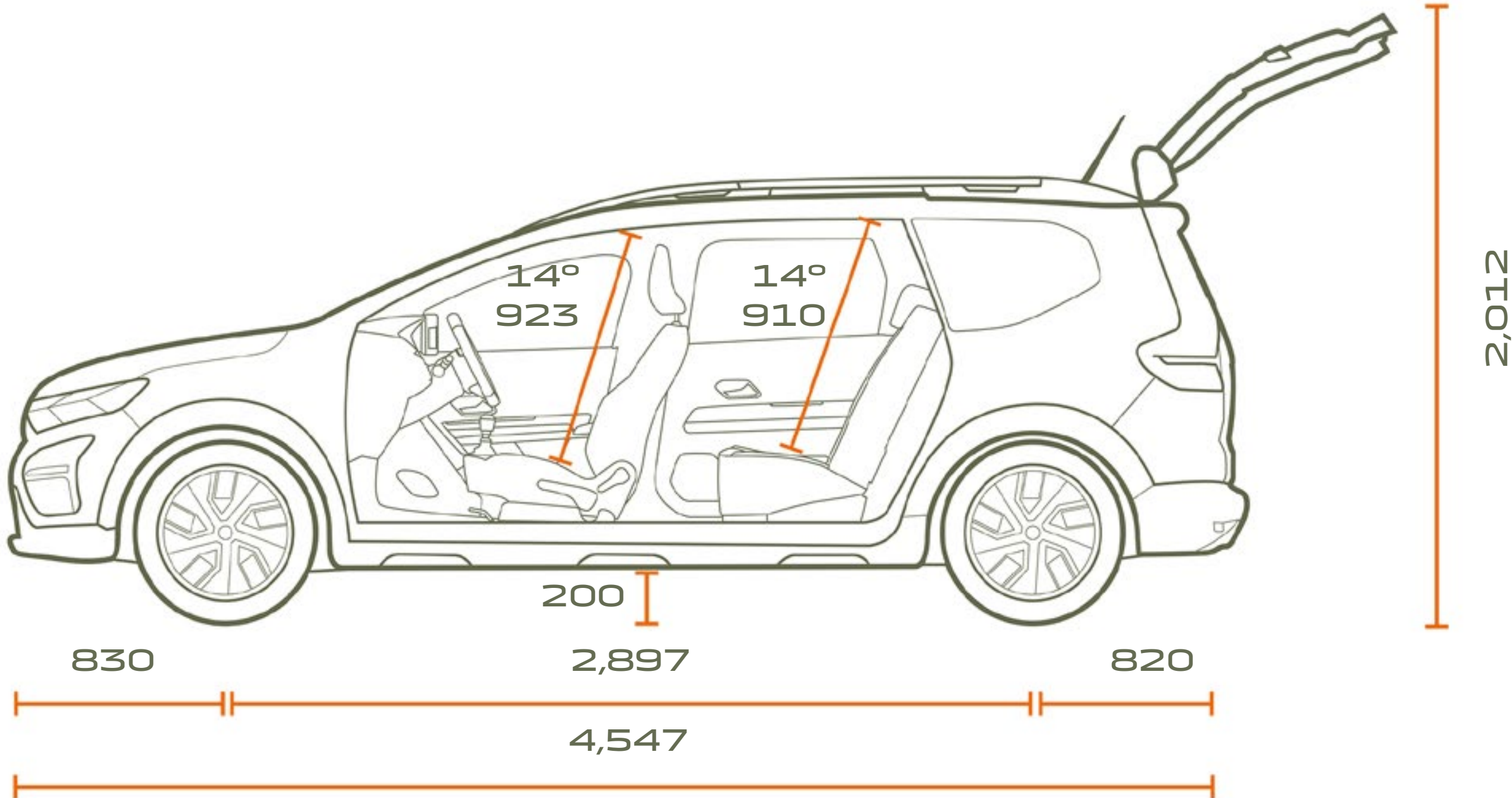
СТРАНИЧЕН ПОГЛЕД НА 5 СЕДИШТА
