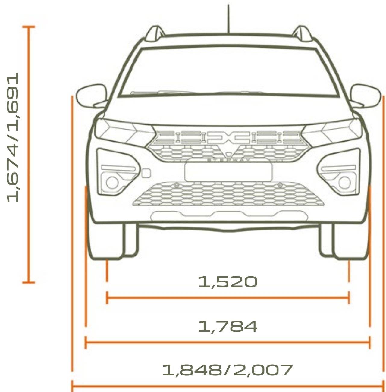
ПРЕДЕН ПОГЛЕД НА 5 И 7 СЕДИШТА
