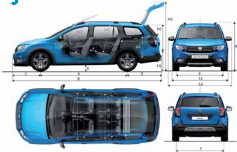
LOGAN MCV PROSTORNINA PRTLJAŽNIKA (dm³) (ISO STANDARD 3832)
