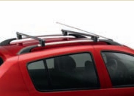
Las barras de techo transversales sobre longitudinales permiten transportar 80 kg de equipaje o instalar otros accesorios.
