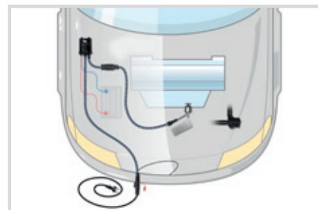
ELEKTRISK MOTORVÄRMARE sänker dina bränslekostnader. Den kopplas till vanligt eluttag och går att styra med timer på elstolpe. Motorvärmaren går att komplettera med kupékontakt och kupévärmare. Paketnummer: VÅ014
